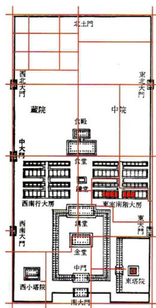
(伽藍図)
