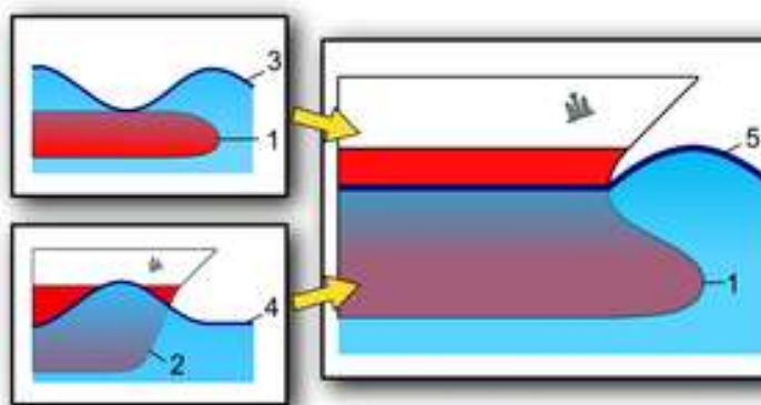
バルバス・バウの効果
